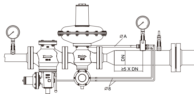
切断阀 + 调压器（内置切断）连接图
