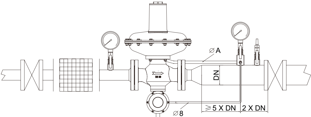
水平位置安装示意图
