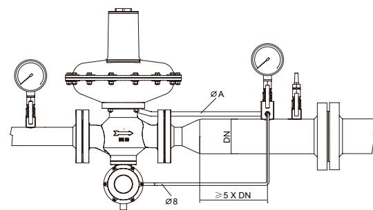
调压器（内置切断）连接图
