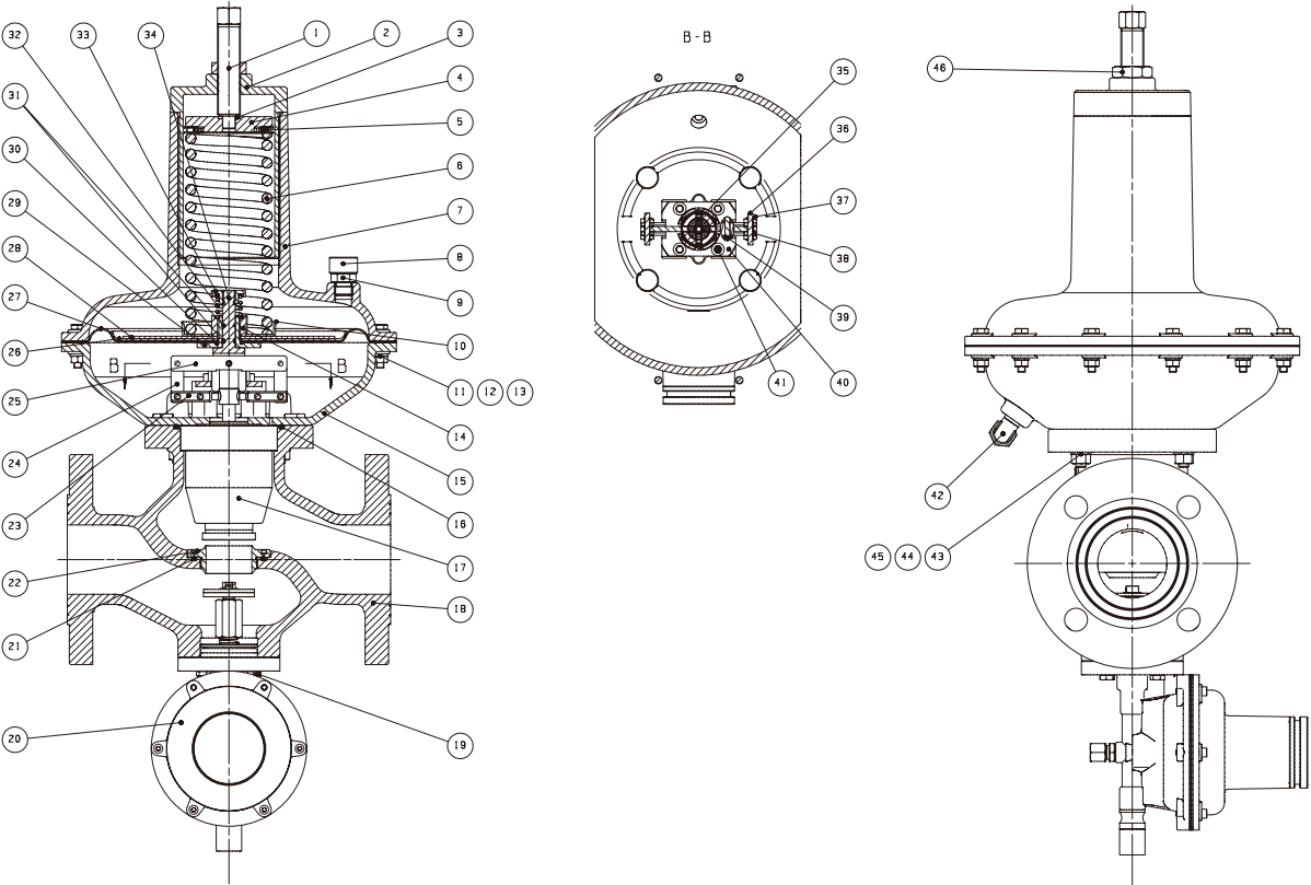
调压器
